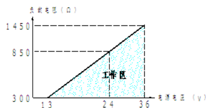
图 10：4-20mA 电流输出负载特性
