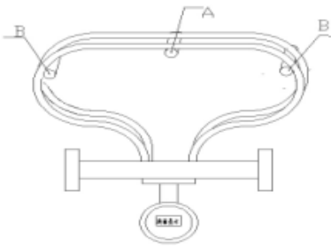
图 2 科里奥利传感器一例 A-驱动线圈 B-检测探头
